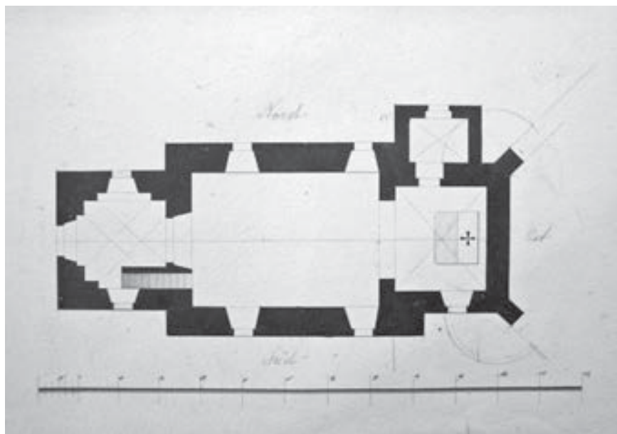
Půdorys kostela ve Starém Místě, 1. polovina 19. století.
