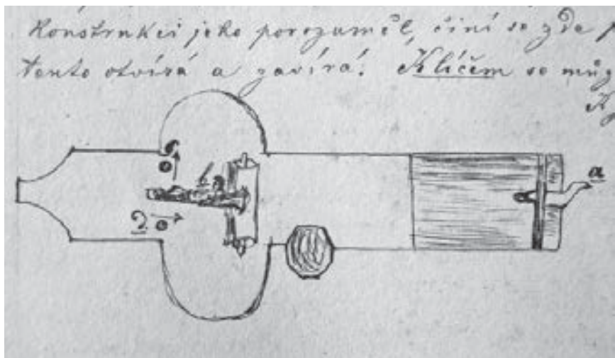
Náčrt zámku na hlavních kostelních dveřích zaznamenaný ve farní kronice.
